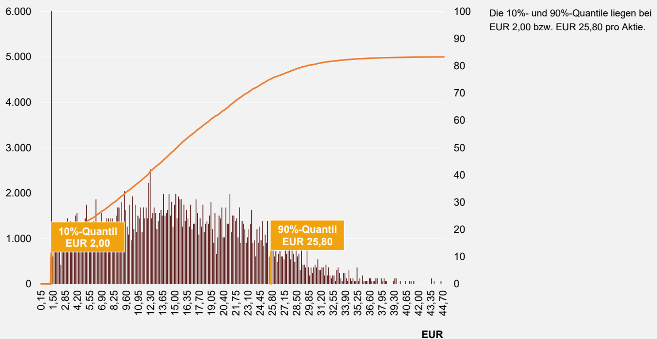
ABBILDUNG 1: MONTE-CARLO-SIMULATION
